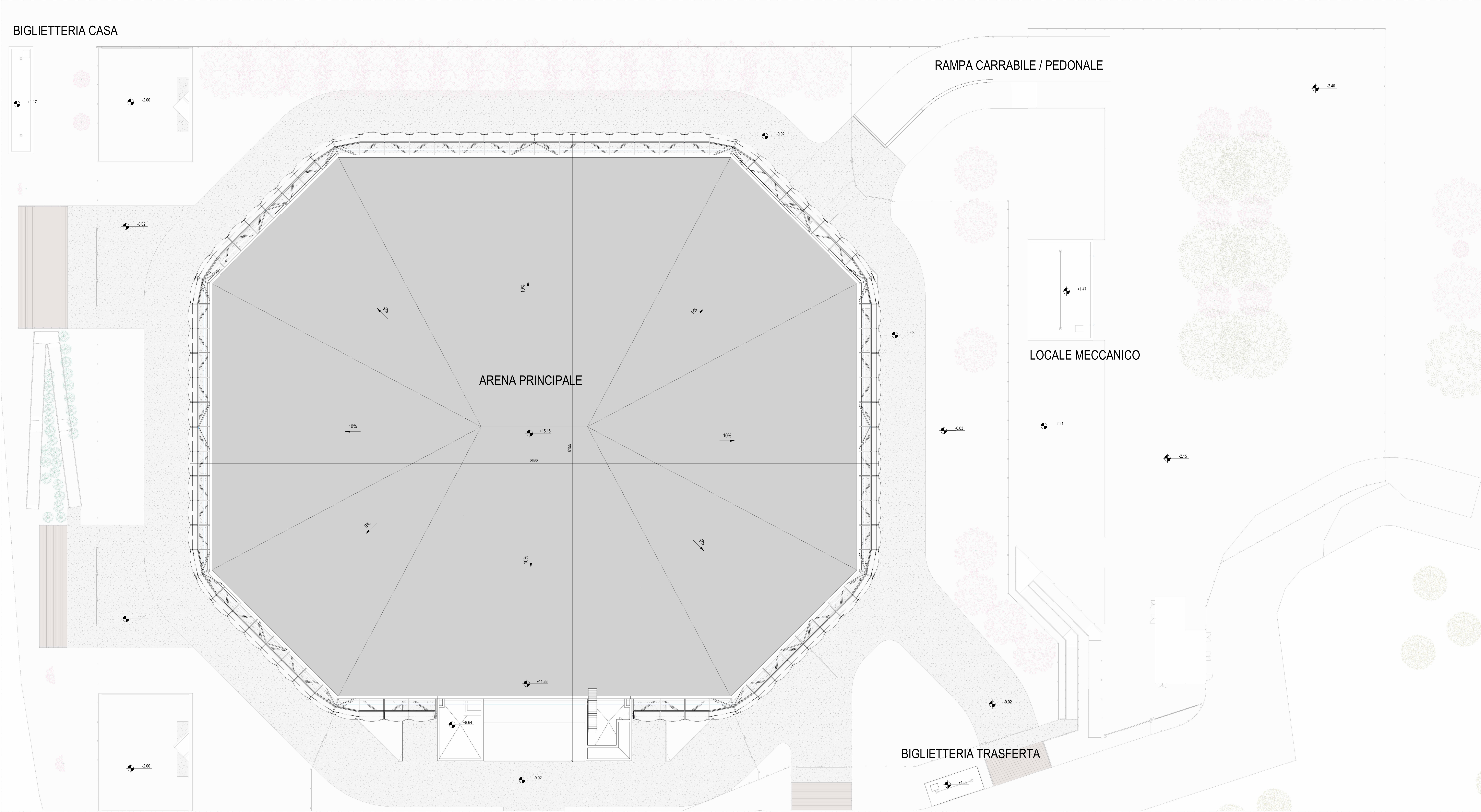
PLANIMETRIA GENERALE 1:200
