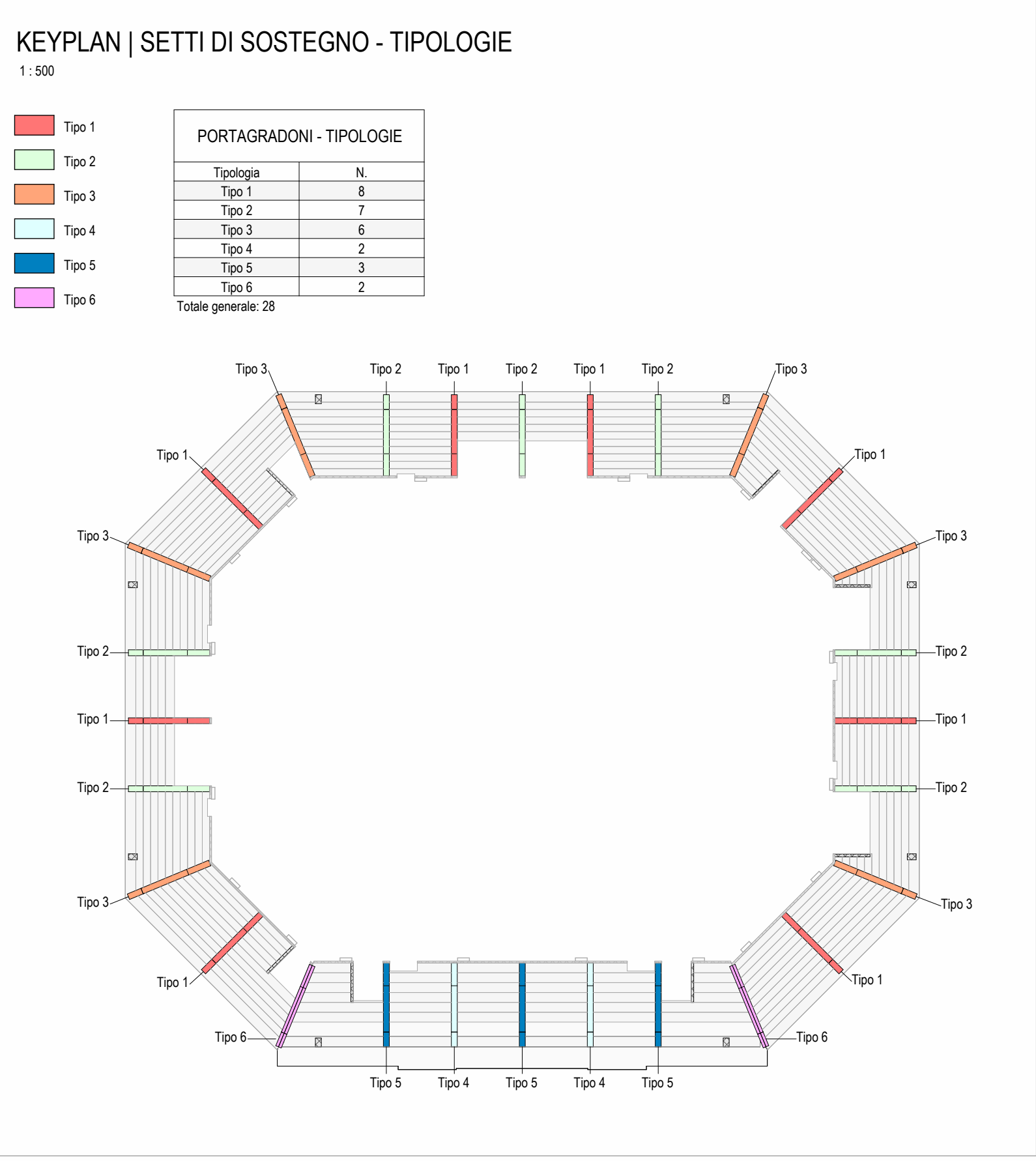
KEYPLAN | SETTI DI SOSTEGNO - TIPOLOGIE
