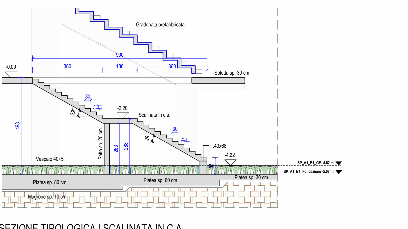
SEZIONE TIPOLOGICA | SCALINATA IN C.A.
