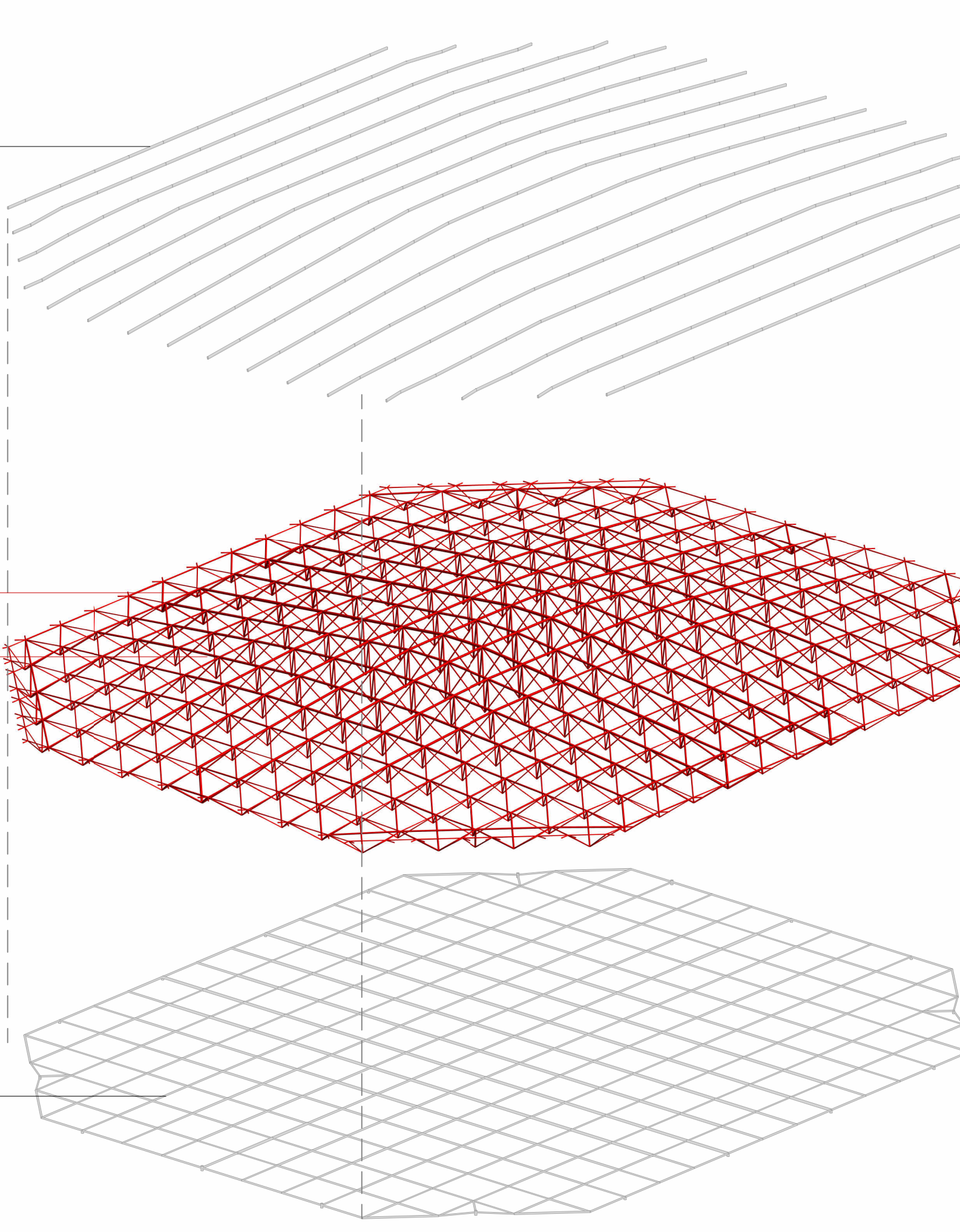
SVILUPPO COPERTURA METALLICA
