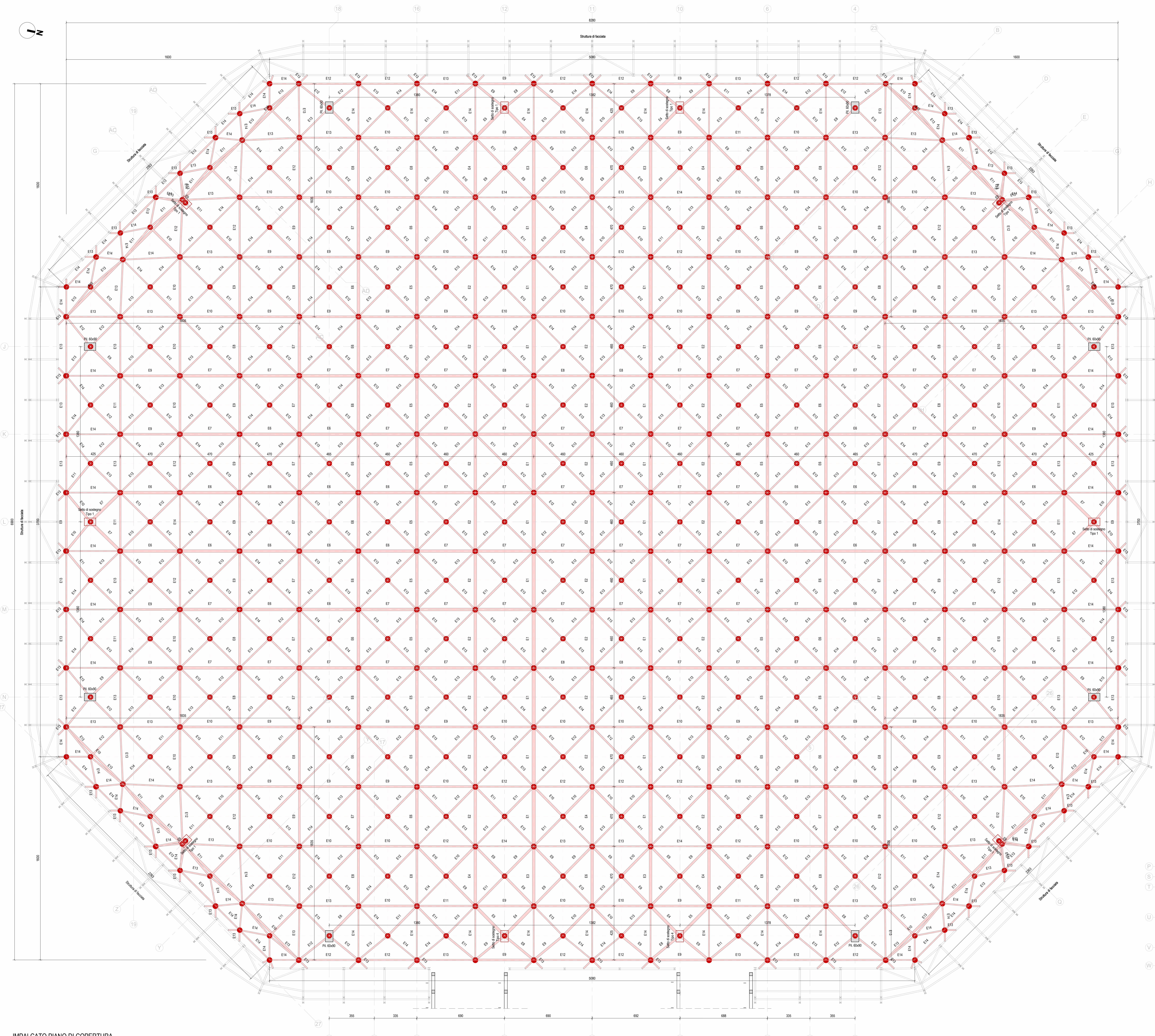
IMPALCATO PIANO DI COPERTURA
