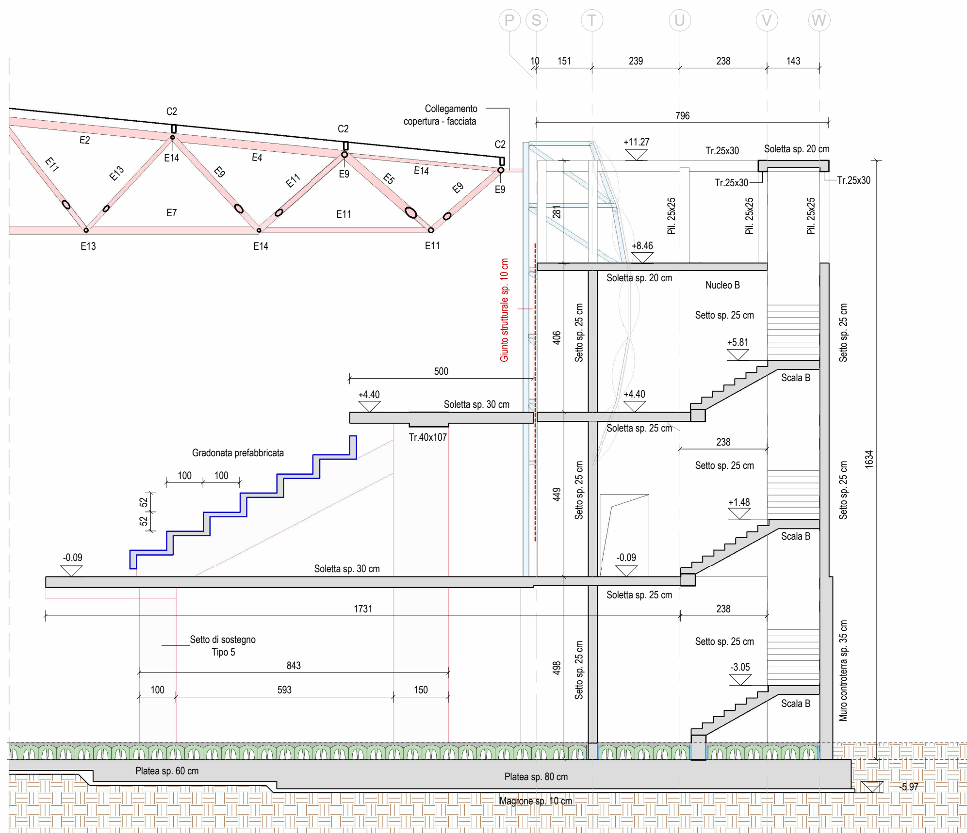
SEZIONE C-C 1: 100
