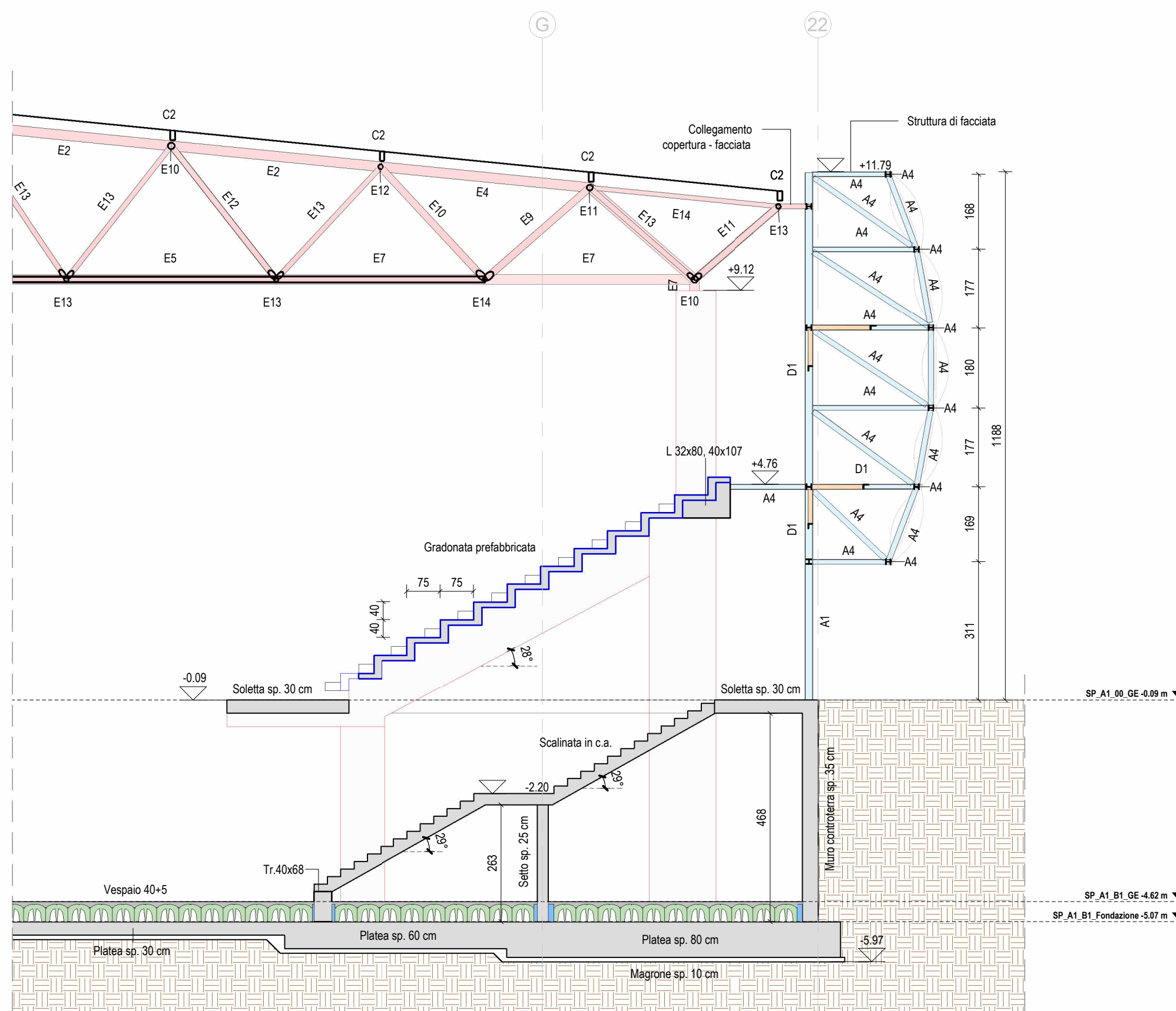
SEZIONE D-D 1: 100
