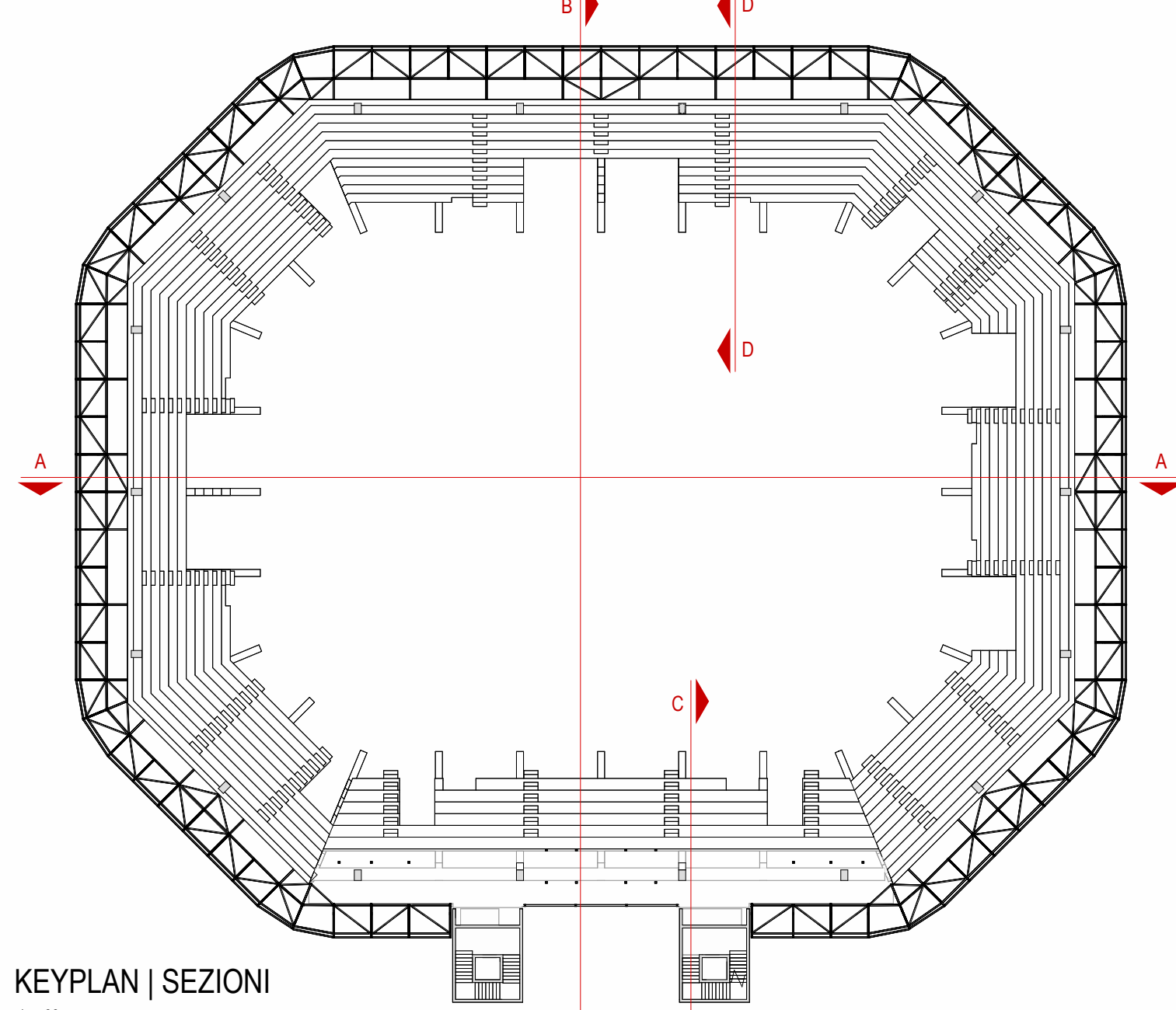
KEYPLAN | SEZIONI 1: 500
