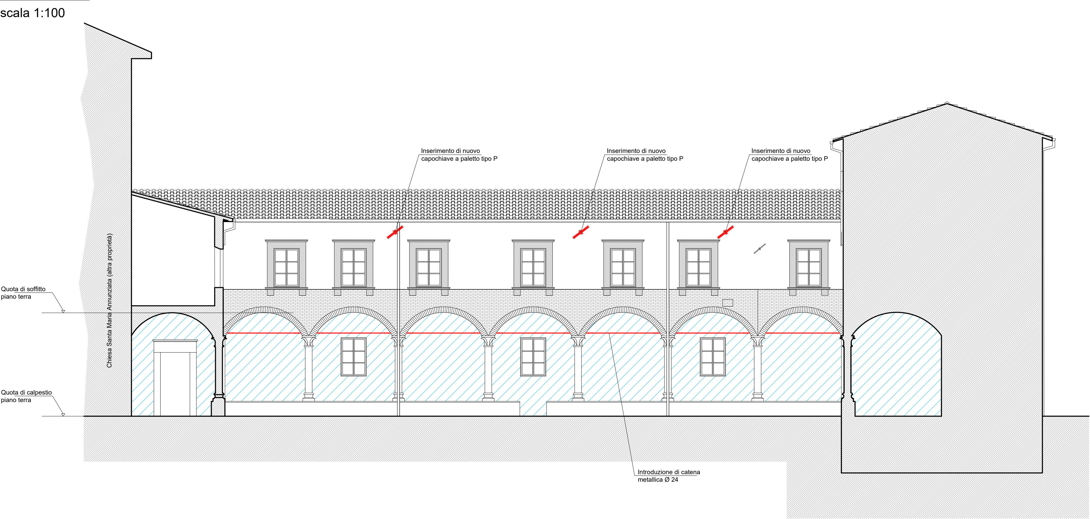
8 - PROSPETTO CHIOSTRO INTERNO
