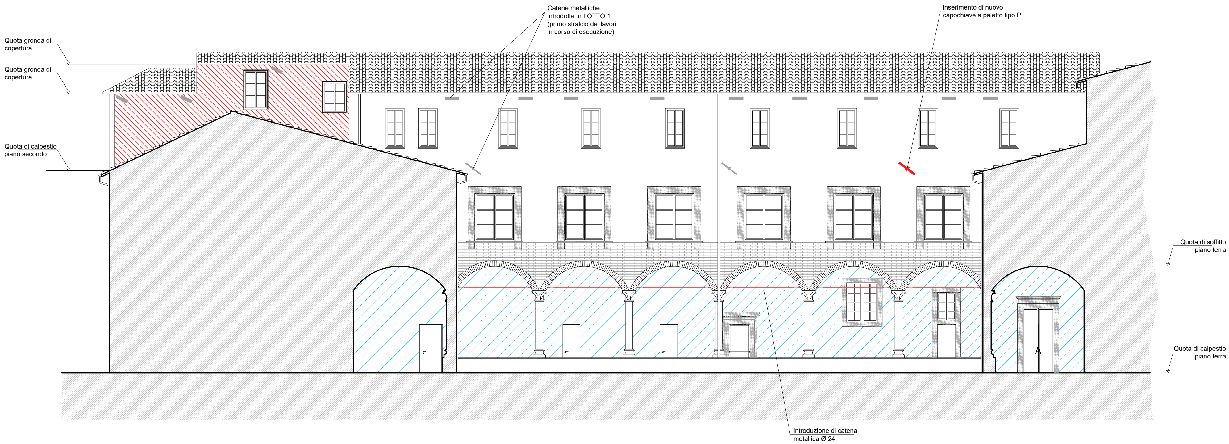
4 - PROSPETTO CHIOSTRO INTERNO
