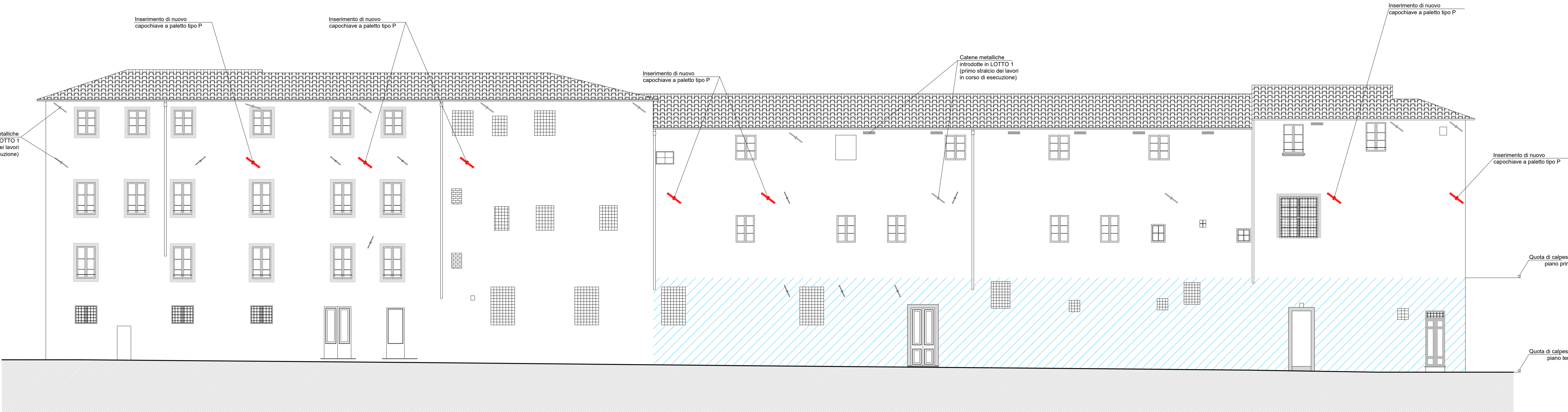
5 - PROSPETTO VIA VALLISNERI
