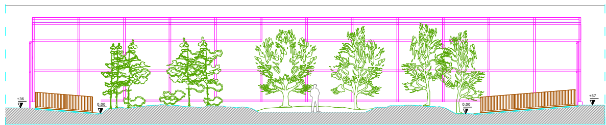
SEZIONE B-B'
