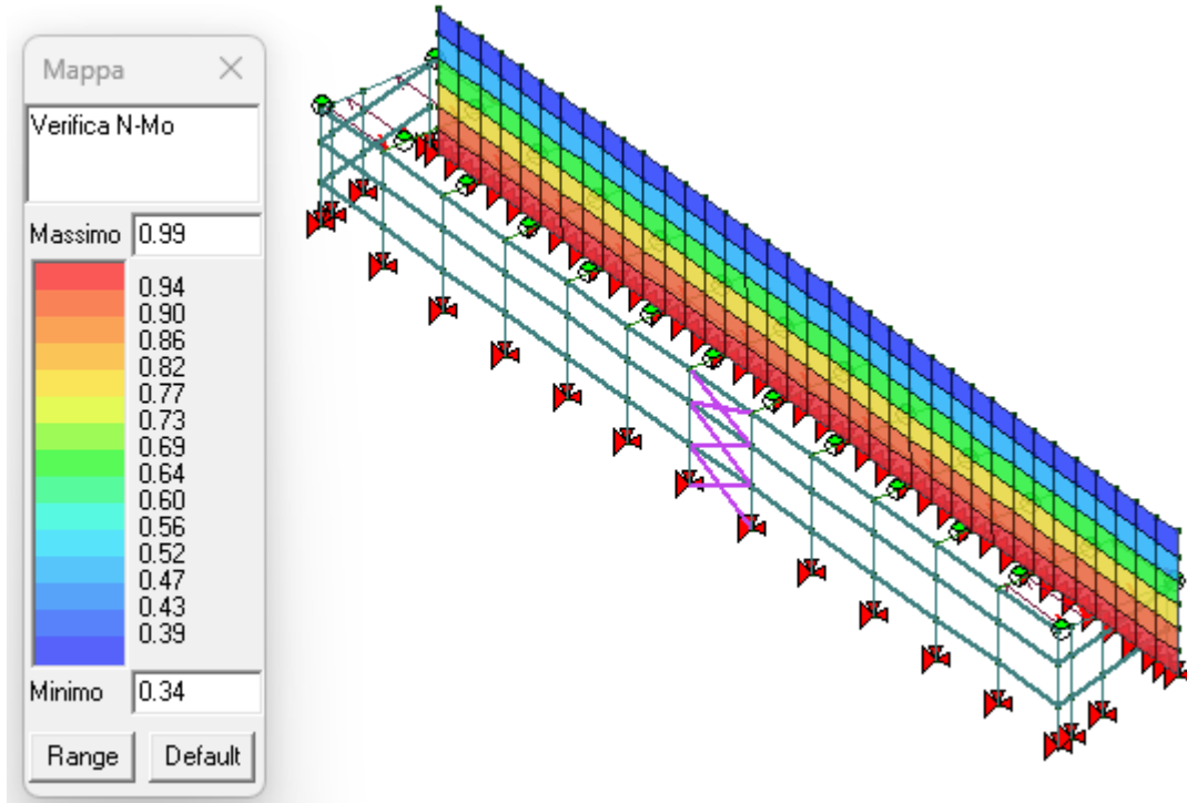
Verifica N-Mo: verifica a pressoflessione fuori dal piano dei maschi murari per le combinazioni con il sisma senza interventi di rinforzo (§7.8.2.2.3 D.M.2018)
