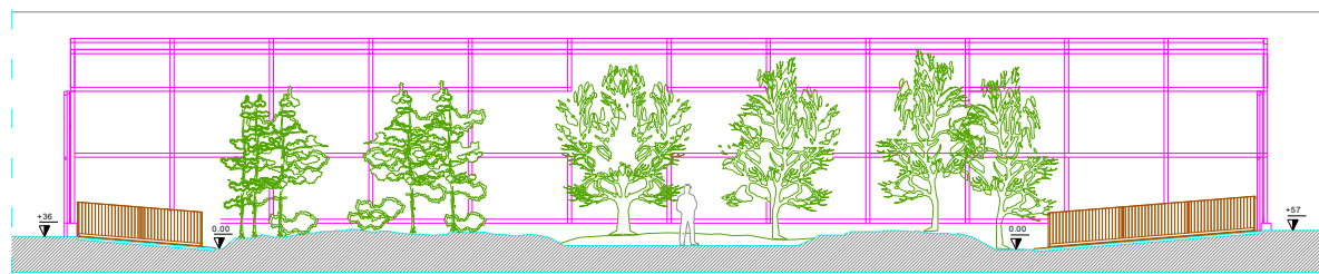
SEZIONE B-B'
