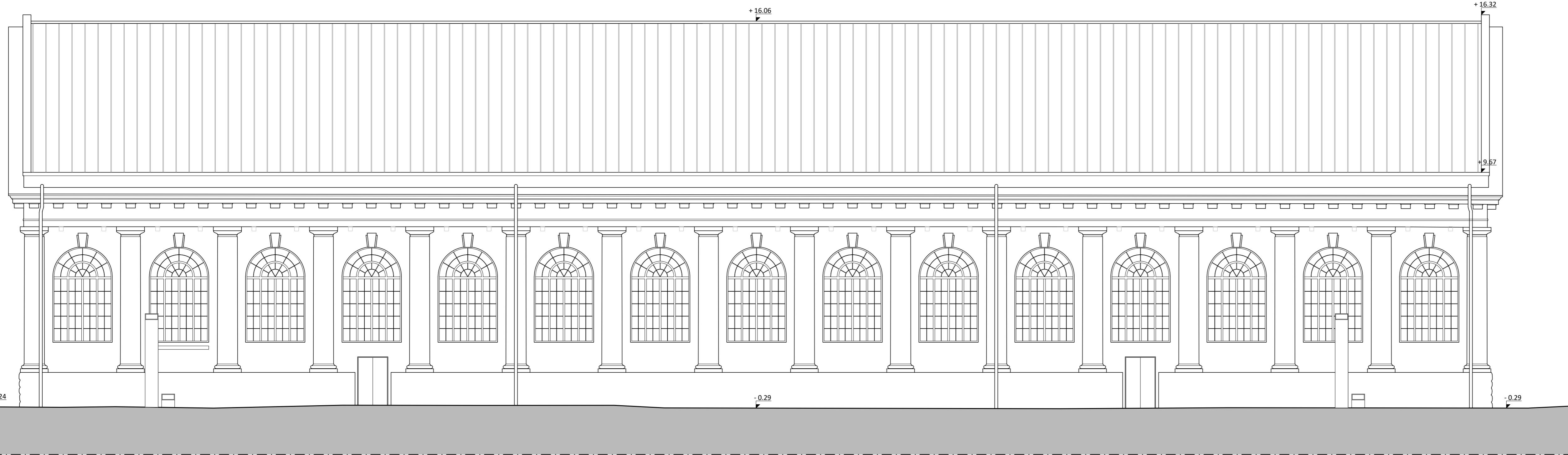
PROSPETTO OVEST
